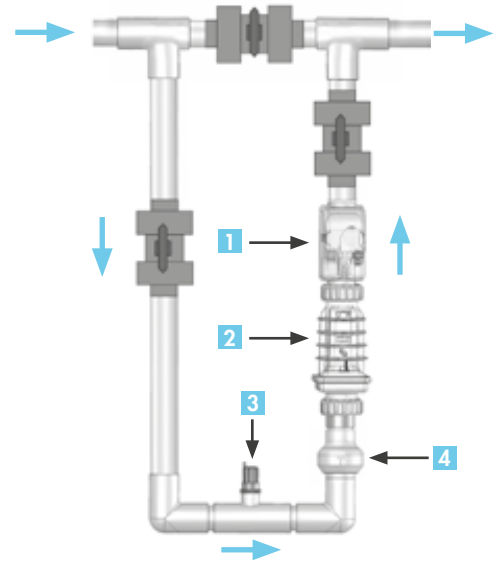
Instalación en U y by-pass
