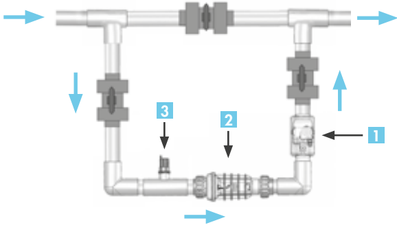
Instalación horizontal y by-pass
